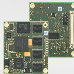
phyCARD-M
